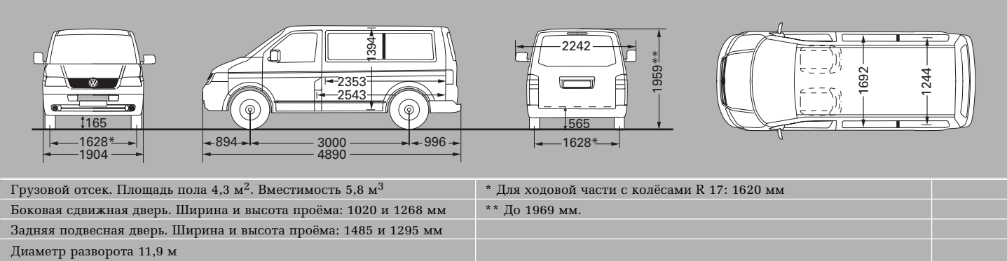
Transporter Kombi, короткая база, средняя крыша
