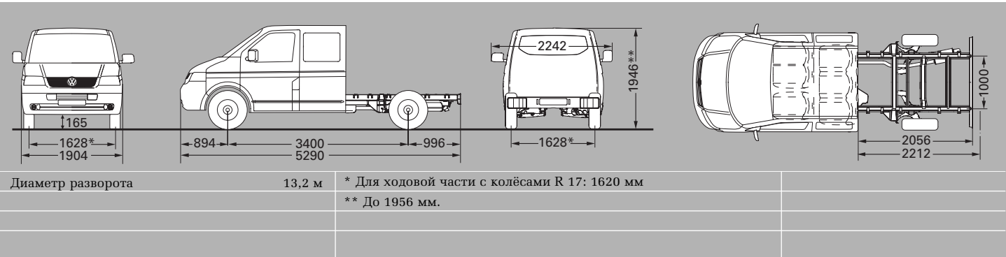
Transporter Шасси, длинная база, со вдвоенной кабиной
