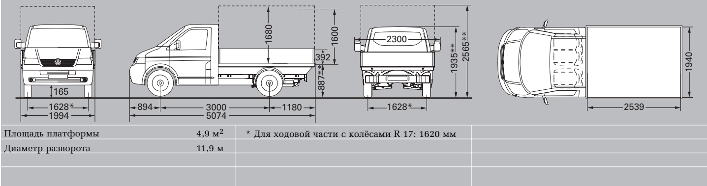
Transporter Pritsche, длинная база с одиночной кабиной
