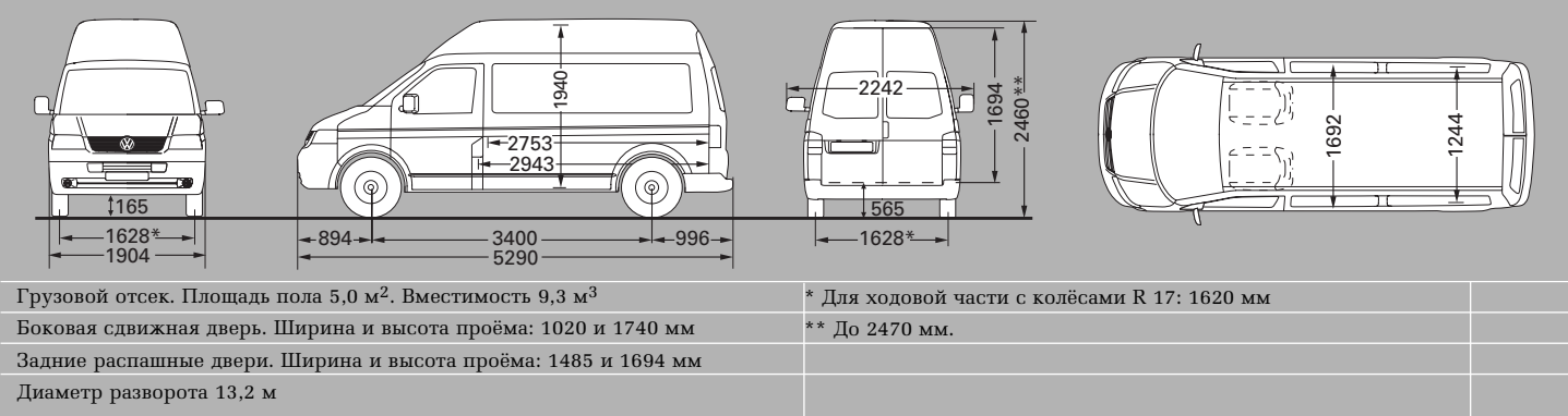
Transporter Kombi, Caravelle, короткая база, стандартная крыша
