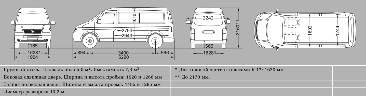
Transporter Шасси, короткая база, с одиночной кабиной
