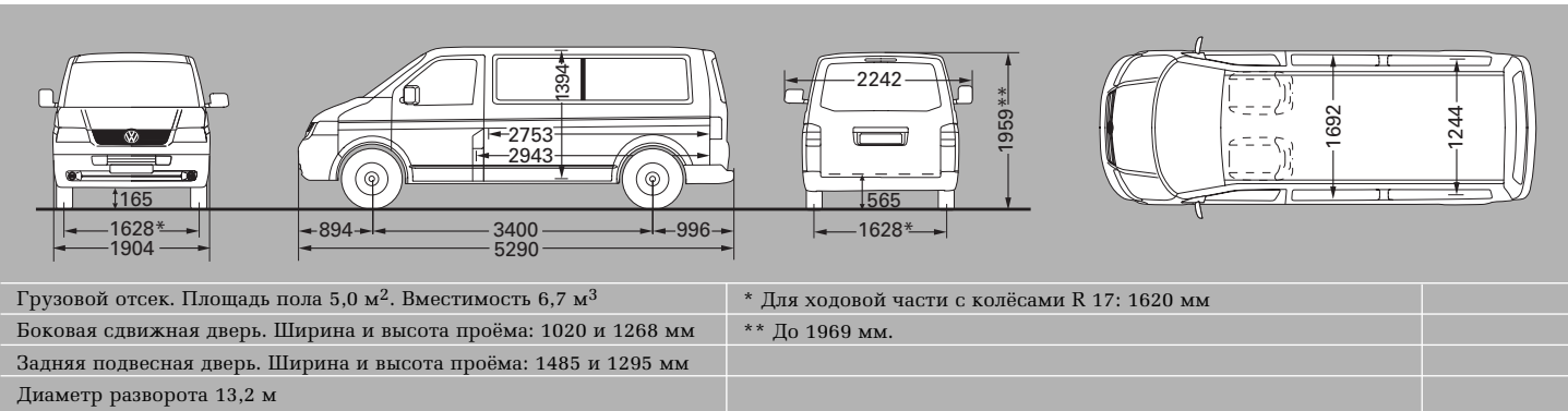
Transporter Kombi, Caravelle, длинная база, стандартная крыша
