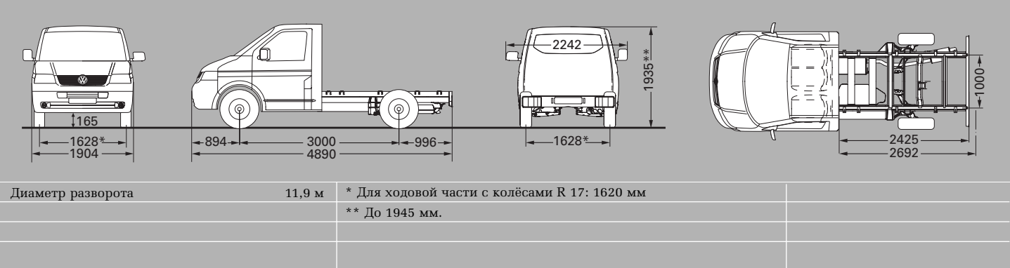
Transporter Шасси, длинная база, с одиночной кабиной
