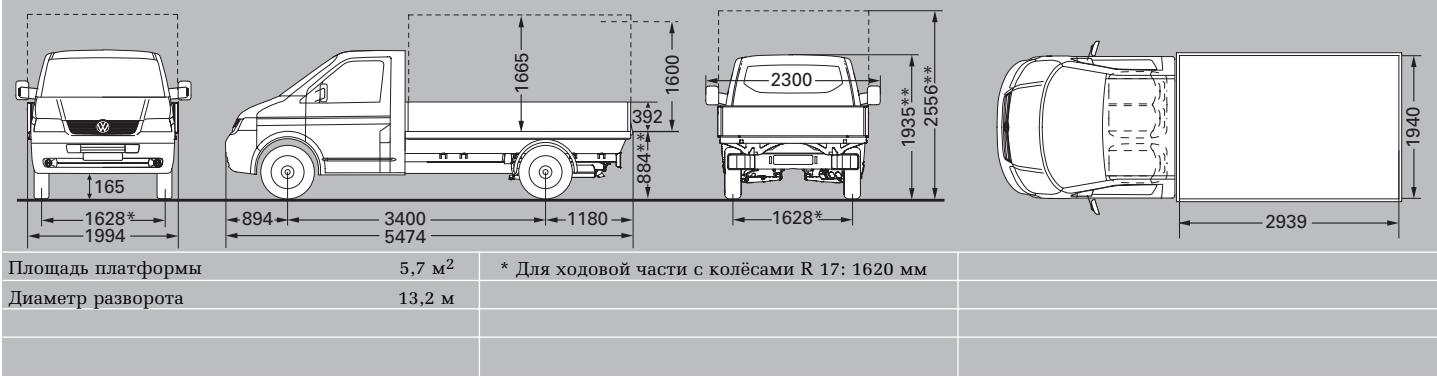
Transporter Pritsche низкопольный, длинная база с одиночной кабиной
